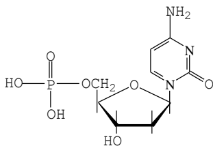
цитозиндезоксирибонуклеотид
