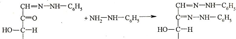
озон глюкозы
