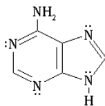
Аденин (6-аминопурин)
