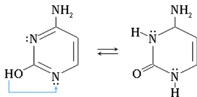
Цитозин (4-амино-2-гидроксипиримидин)
