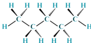
Стереохимическая формула
